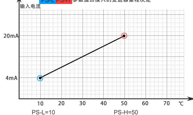
电流输入: 电流信号对应仪表显示
