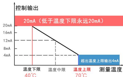
4-20mA上下限控制加热（线性调节）
