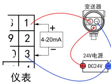
三线制4-20mA接线方式:
